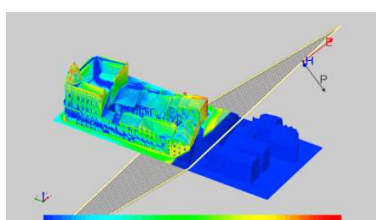
Simulation électromagnétique d'un quartier de ville
